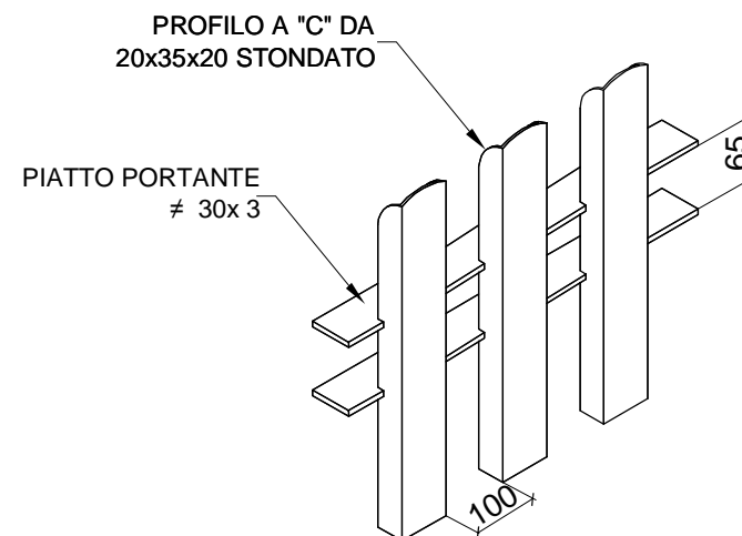
Vista assonometrica
